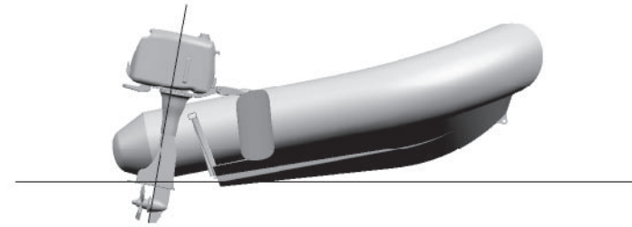
Bug oben, zu viel Trimm nach außen
