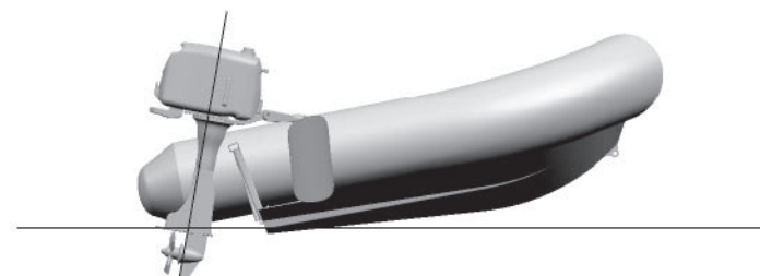
L'avant du bateau déjàuge, trop de trim positif
