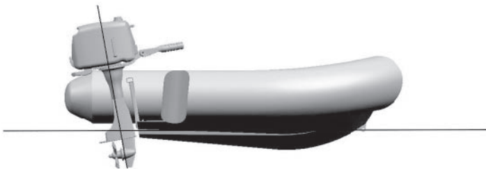
Bug unten, zu viel Trimm nach innen
